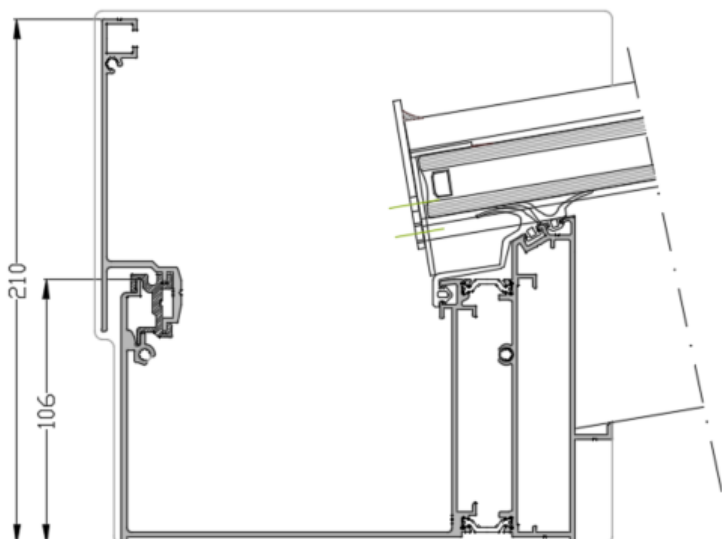
Chéneau carré avec VER130
