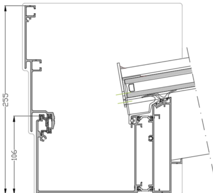
Chéneau carré avec VER121
